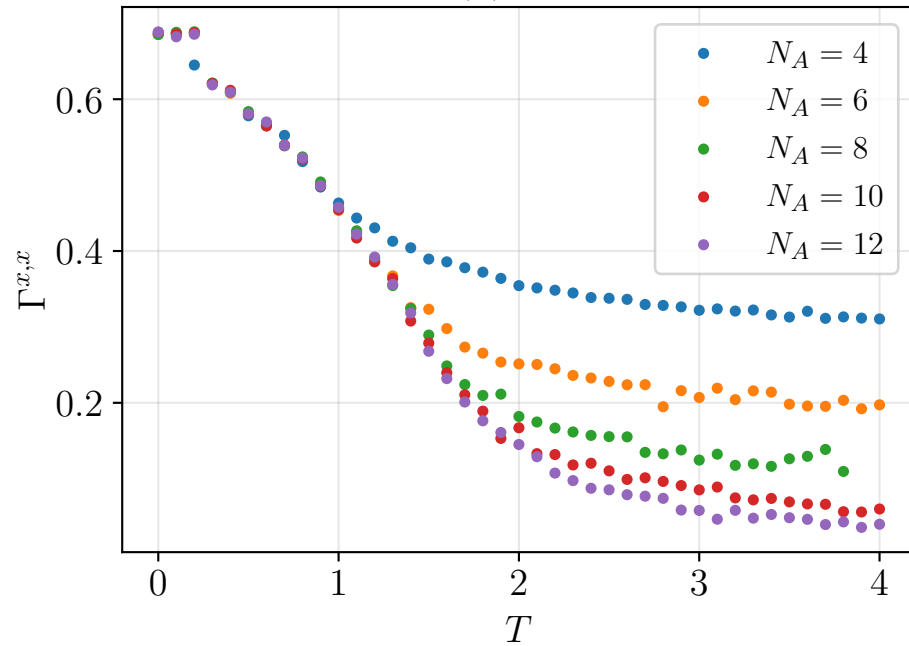
(b) \Gamma^{x,x}
