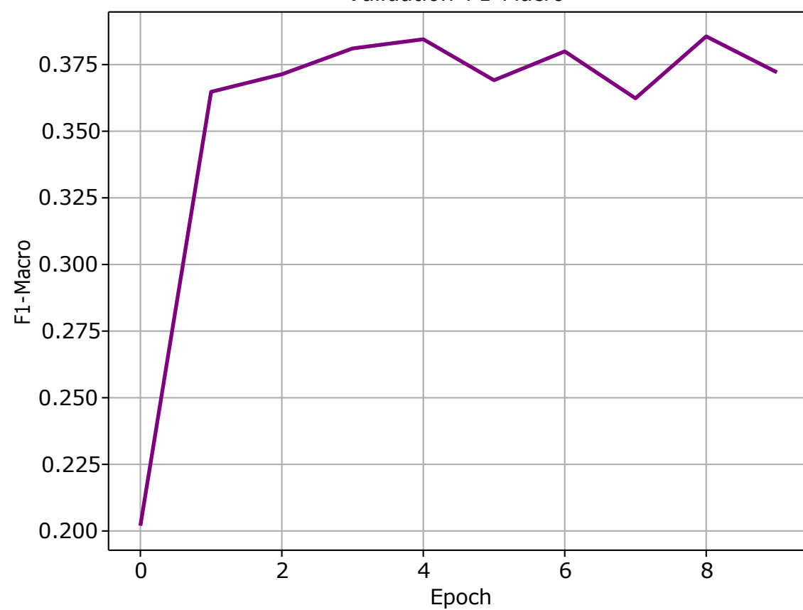
Validation F1-Macro
