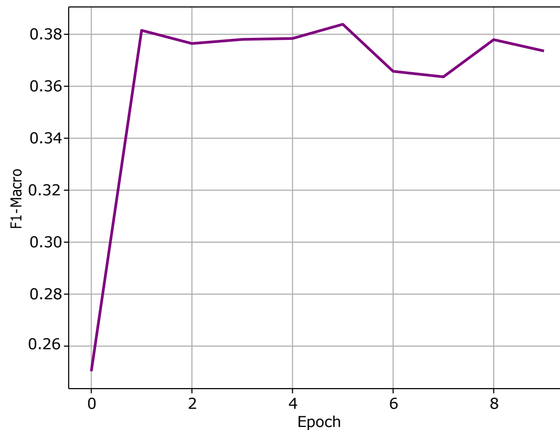
Validation F1-Macro
