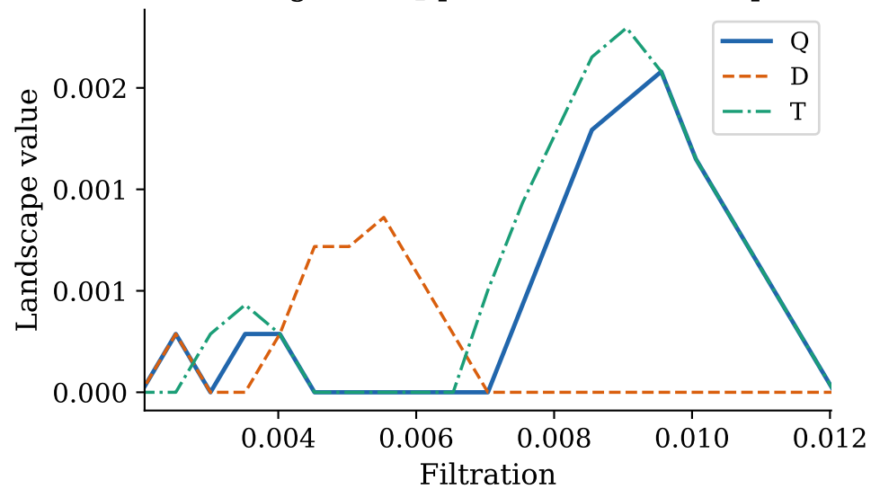
(D) Weighted H_1 persistence landscapes
