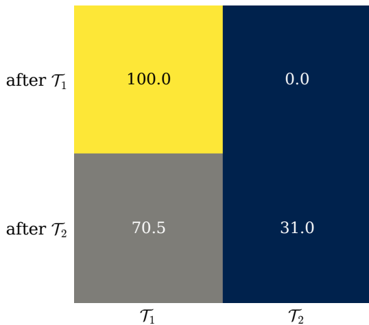
(d) EWC+Replay
