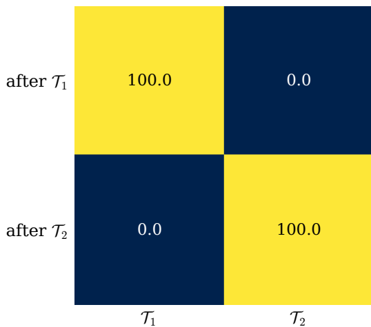
(b) EWC
