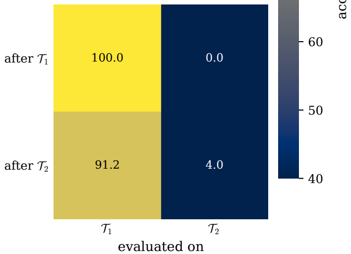
(d) EWC+Replay ( \lambda = 500 )
