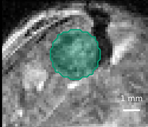
SAM2 prompt
