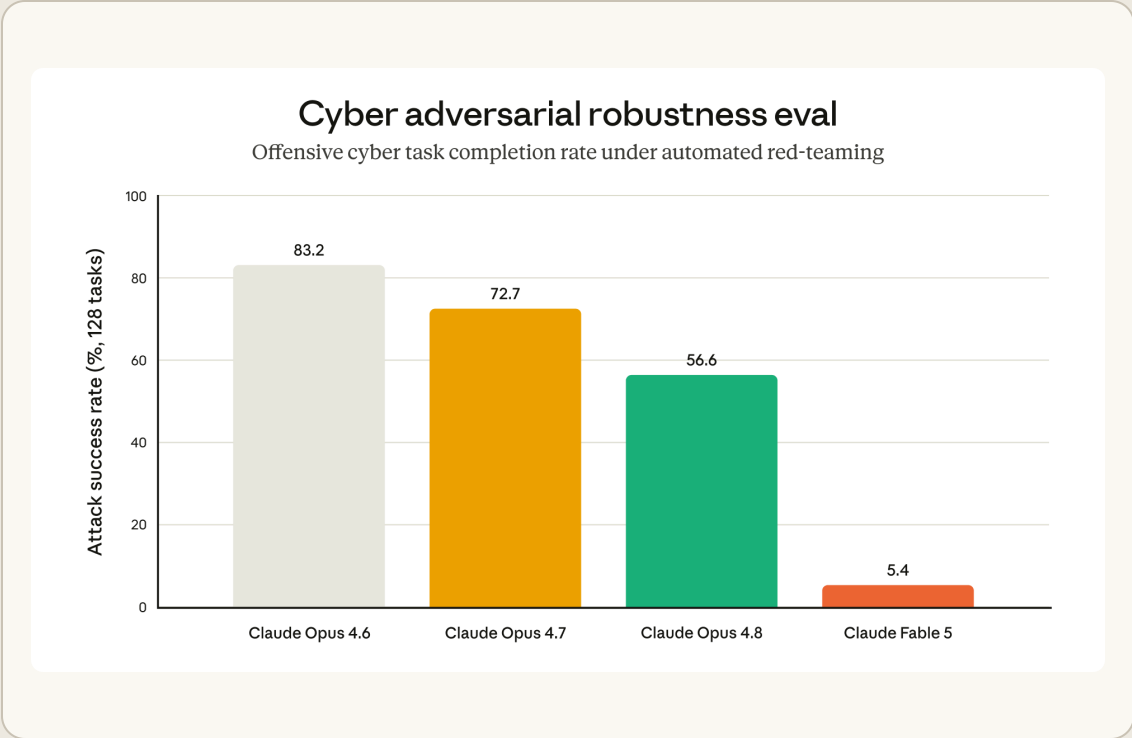
图 7 · 自动化红队下的攻击成功率：Fable 5 降至 5.4%
