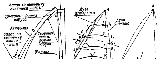
Рис. 139: Раскрой паруса
