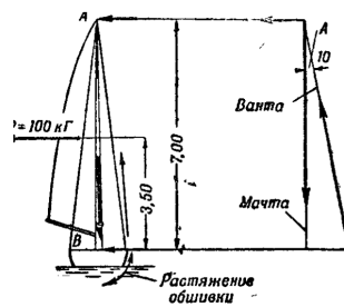
Рис. 158: Силы, действующие на мачту и ванта
