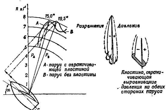
Рис. 111: Влияние ограничивающей пластины на аэродинамическую силу паруса
