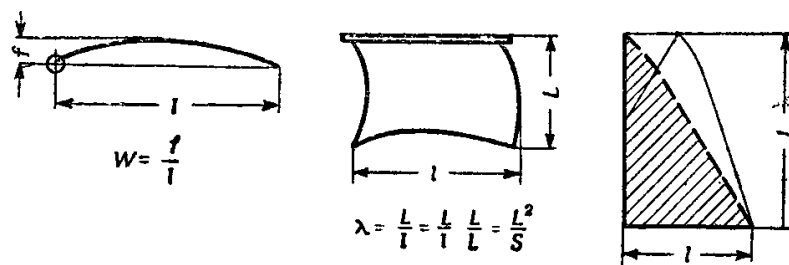
Рис. 62: Удлинение и пухатость паруса: W = f/l ; \lambda = L/l = L^2/S
