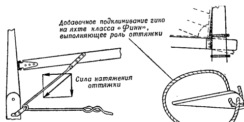
Рис. 85: Оттяжка гика и дополнительное подкливание гика на яхте класса «Финн»
