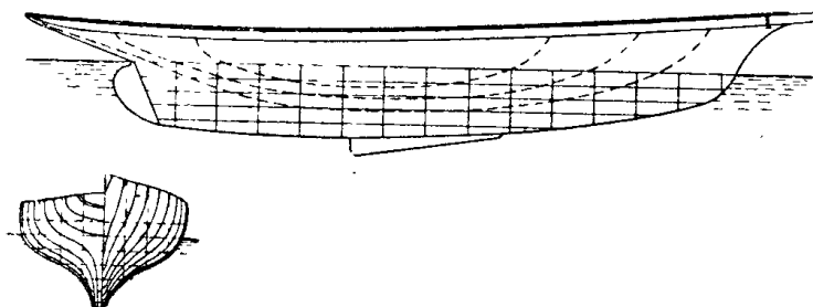
Рис. 29: Яхта «Волонтер»
