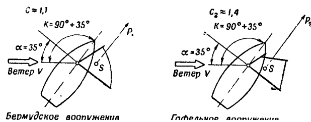
Рис. 113: Сравнение аэродинамических сил бермудского и гафельного парусов на курсе бакштаг
