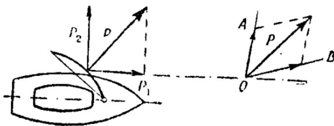
Рис. 7: Разложение сил
