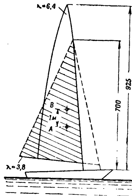
Рис. 112: Яхта с двумя вариантами парусов различной удлинённости
