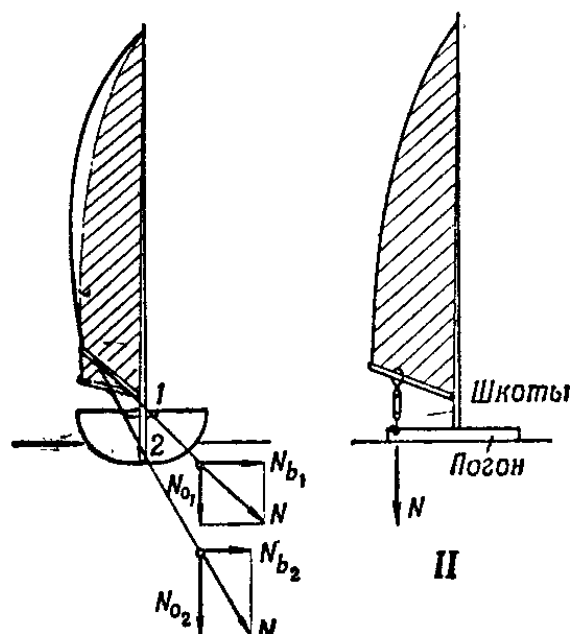
Рис. 91: Влияние места крепления шкотов на перекручивание паруса
