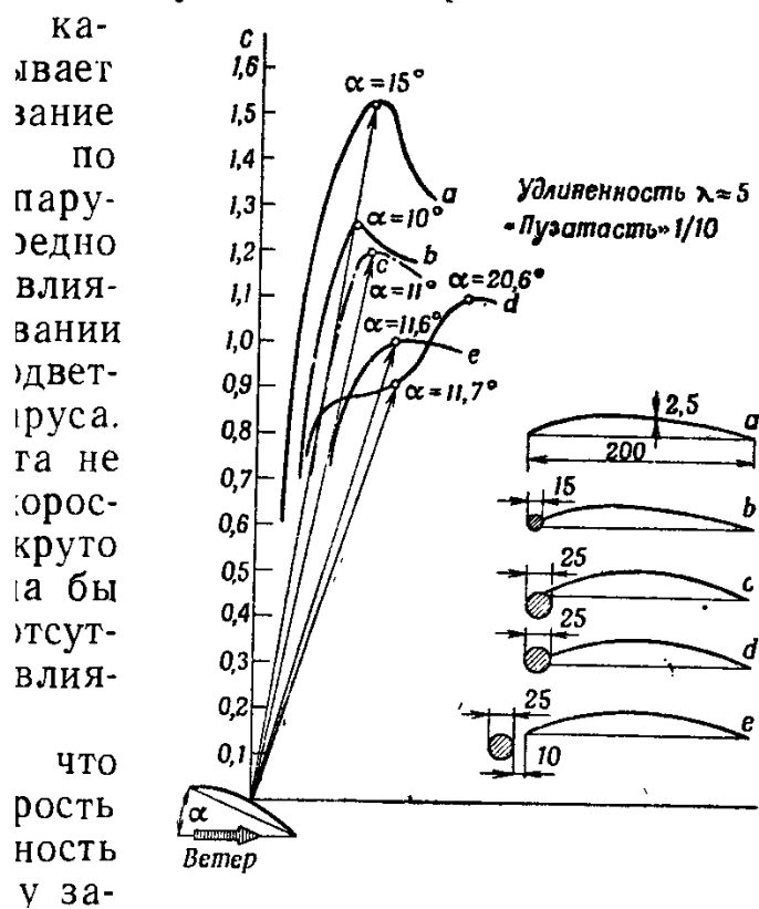
Рис. 115: Зависимость коэффициента C от угла атаки при различном расположении и величине мачты
