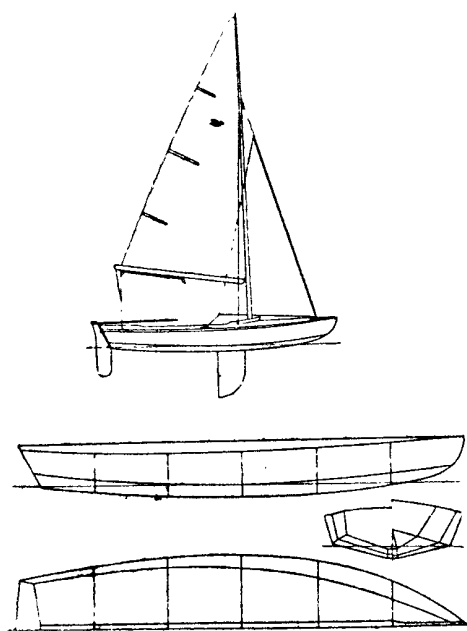
Рис. 39: Швертбот «Снайп»
