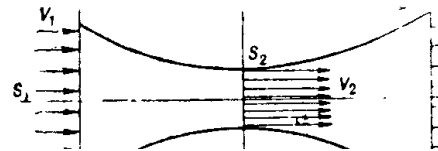
Рис. 53: Труба переменного сечения
