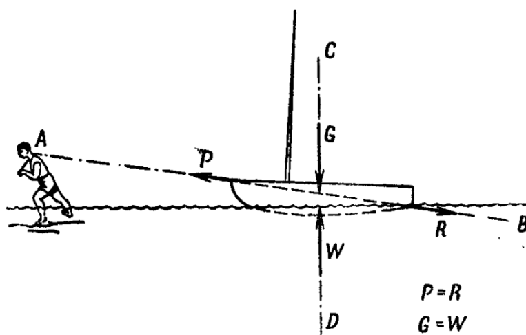
Рис. 2: Буксирование яхты
