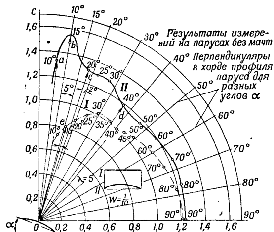
Рис. 66: Полярные кривые аэродинамических коэффициентов: I — \lambda = 5 , W = 1/10 ; II — результаты измерений на парусах без мачт. Перпендикуляры к хорде профиля паруса для разных углов \alpha
