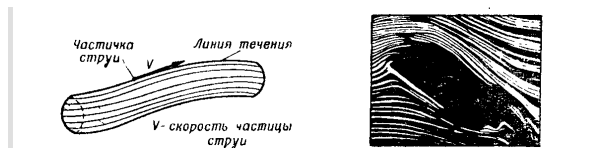
Рис. 52: Струя жидкости: частица струи, линия течения, V — скорость частицы струи
