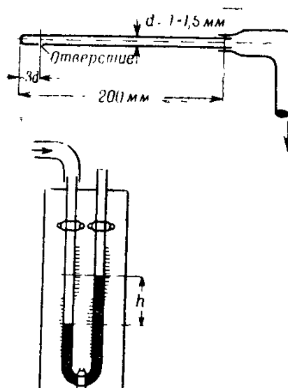
Рис. 61: Аэродинамический лот
