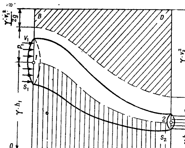
Рис. 54: Графическая иллюстрация уравнения Бернулли
