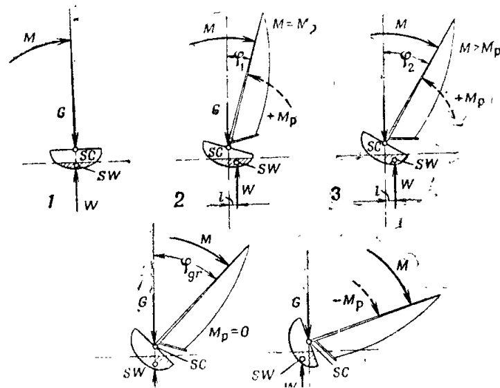
Рис. 14: Крен швертбота
