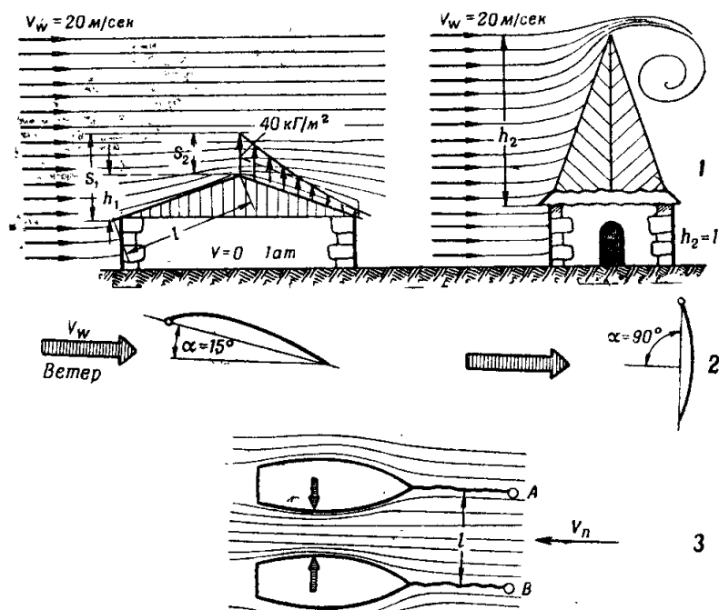
Рис. 51: Примеры действия воздушного и водного потоков: 1 — две крыши; 2 — два паруса; 3 — две лодки на буйках
