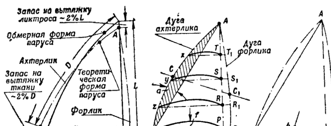
Рис. 139: Раскрой паруса
