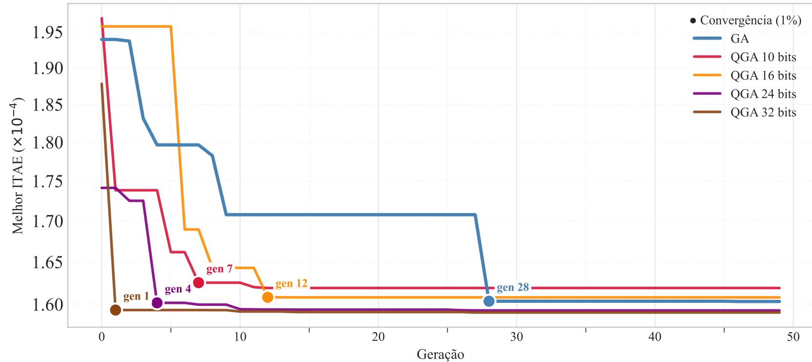
Análise de Convergência: GA vs. QGA (Controlador IT2-FLC)
