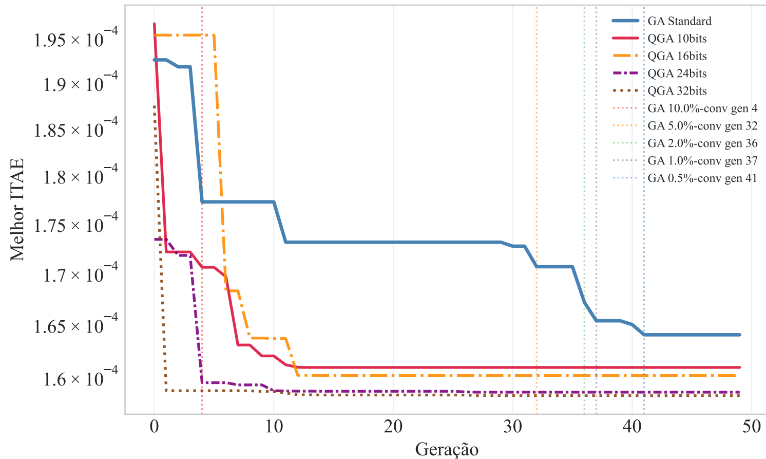
Controlador T1
