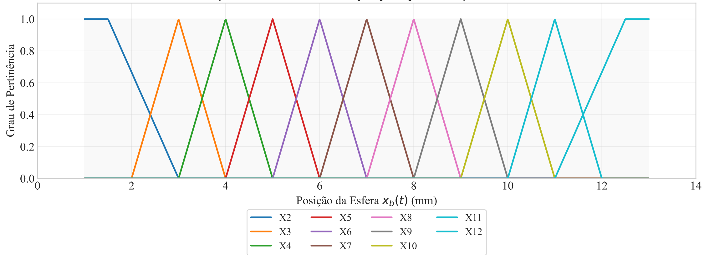
Funções de Pertinência Fuzzy Tipo-1 para Posição da Esfera
