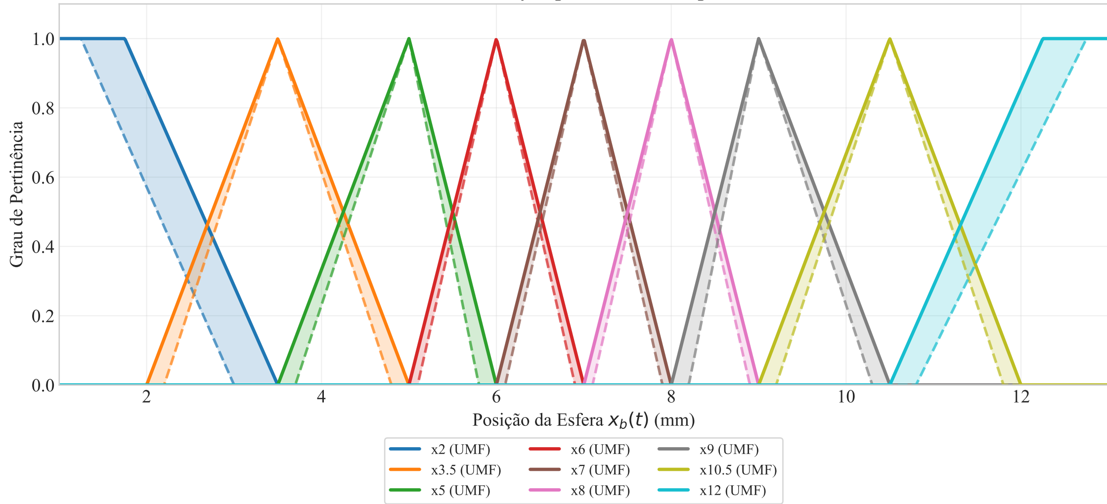
Funções de Pertinência Fuzzy Tipo-2 Intervalar para Posição da Esfera
