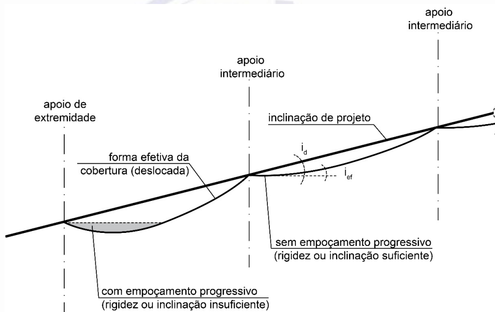
Figura D.1 – Fenômeno do empoçamento progressivo
