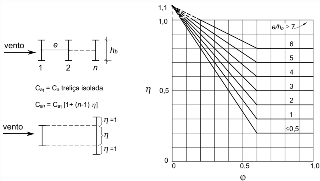
Figura 14 – Fator de proteção \eta para dois ou mais reticulados planos paralelos igualmente afastados
