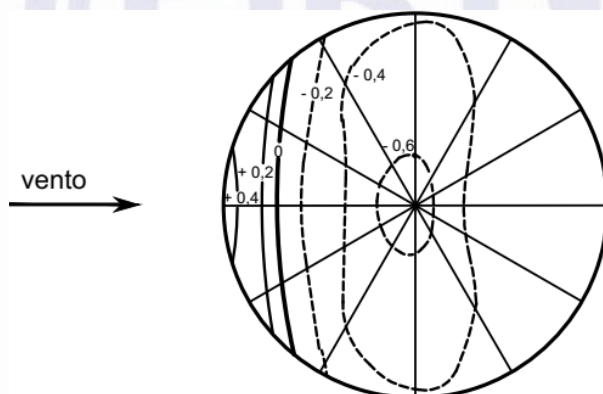
c) Vista superior – Linhas isobáricas dos coeficientes de pressão externa para f/d = 1/4
