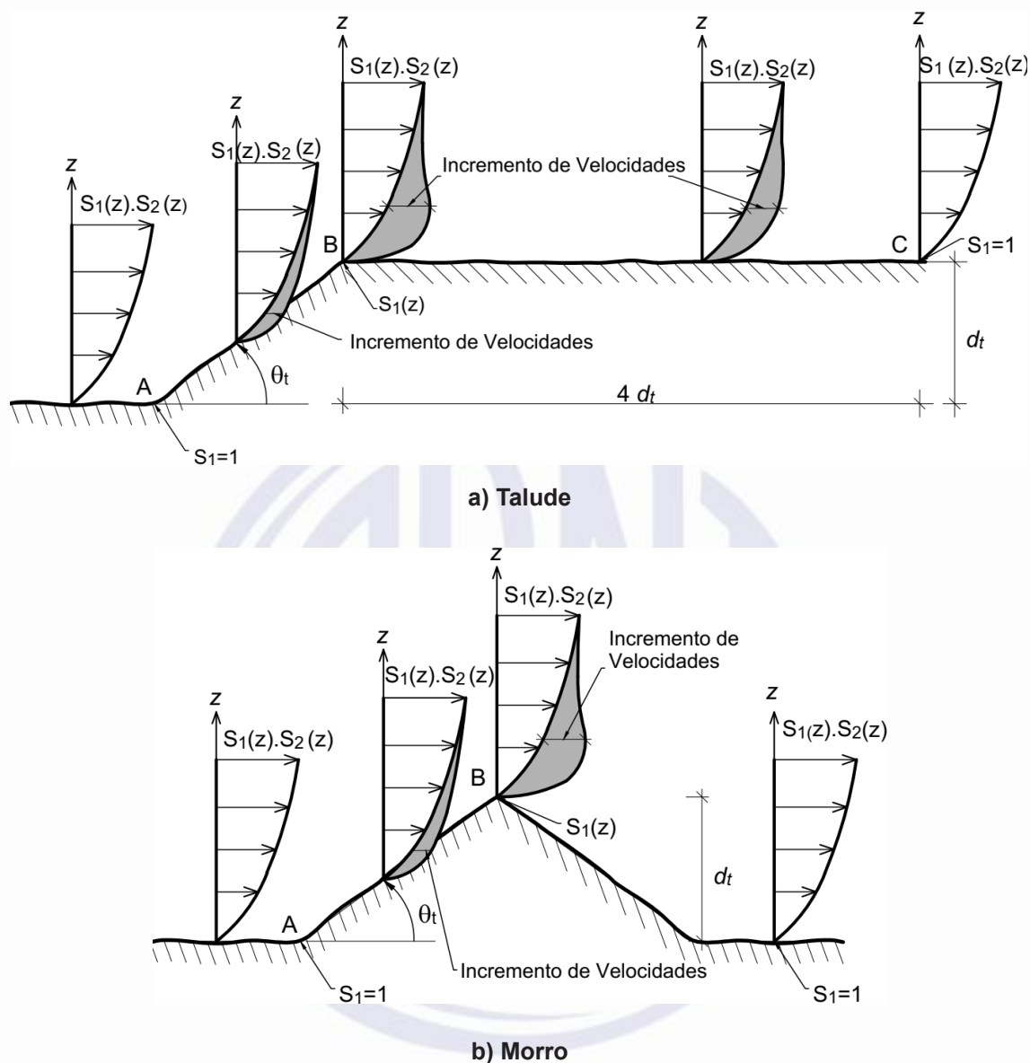
Figura 2 – Fator topográfico S_1(z)
