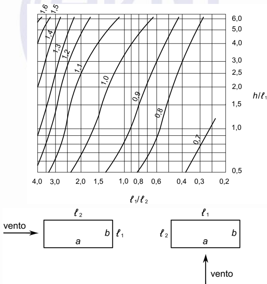
Figura 5 – Coeficiente de arrasto C_a para edificações paralelepípedicas em vento de alta turbulência
