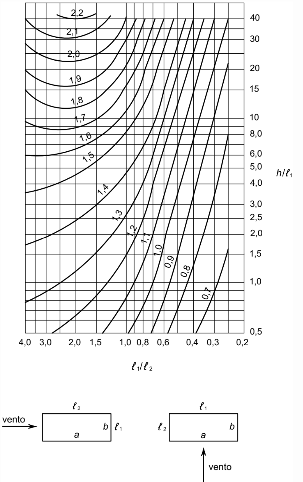
Figura 4 – Coeficiente de arrasto C_a para edificações paralelepípedicas em vento de baixa turbulência
