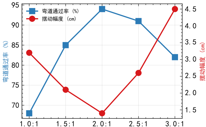
(b) 差速比对循迹性能的影响
