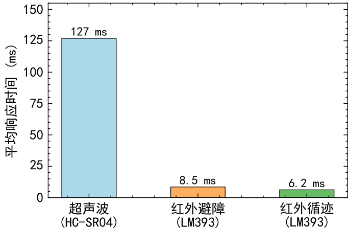
图10 各传感器响应时间对比
