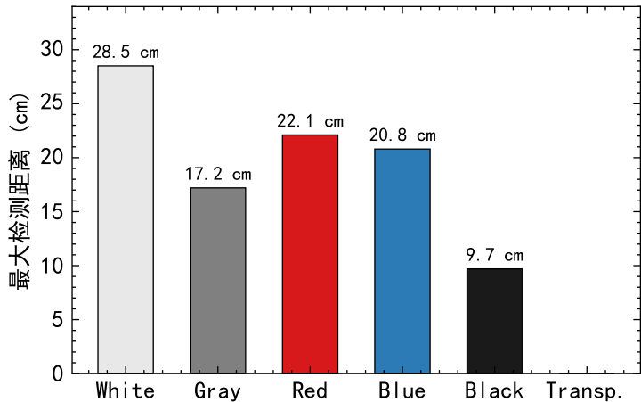
图2 红外避障模块颜色感知特性
