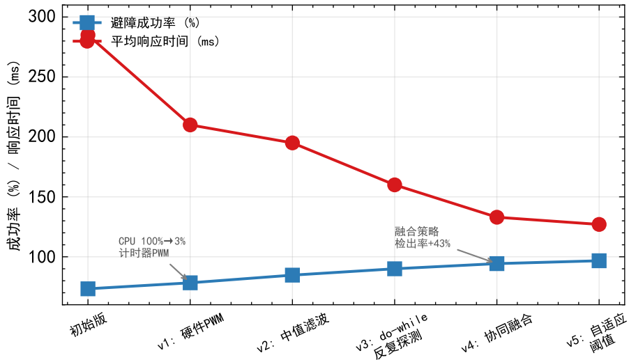
图4 系统性能优化迭代历程
