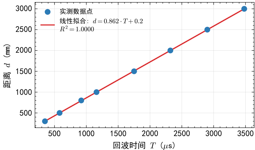
图8 超声波回波时间-距离线性关系
