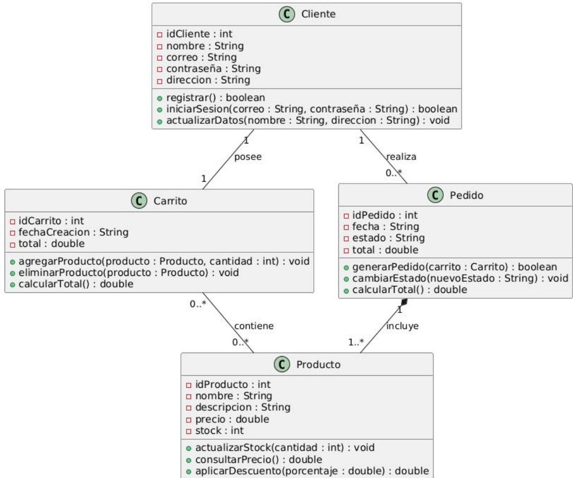
Diagrama de Clases - Sistema Tienda en Línea
