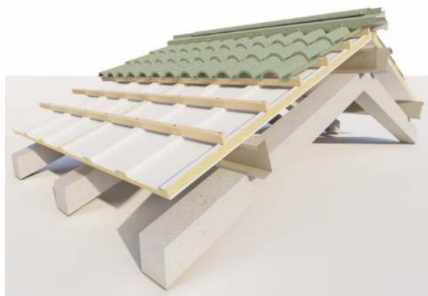
Render ilustrativo — sistema construtivo VENTROOF SYSTEM™
