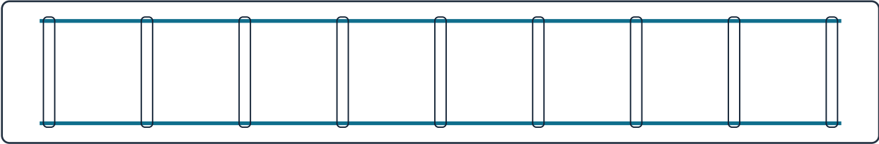
2HA12 sup. + 2HA14 inf. - cadres HA6 / 20 cm
