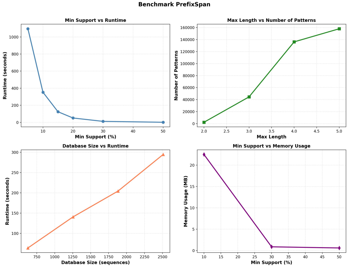
FIGURE 21 – Benchmark de PrefixSpan selon quatre axes. Haut-gauche : décroissance exponentielle du temps d'exécution avec le support minimum ; le coude à 15% justifie notre seuil. Haut-droite : explosion combinatoire du nombre de motifs avec la longueur maximale ; le saut entre 2 et 3 (facteur \times 22 ) est le plus critique. Bas-gauche : scalabilité quasi linéaire avec la taille de la base de séquences. Bas-droite : empreinte mémoire en chute libre au-delà de 20% de support.
