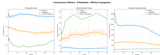
Scores de Silhouette par algorithme
