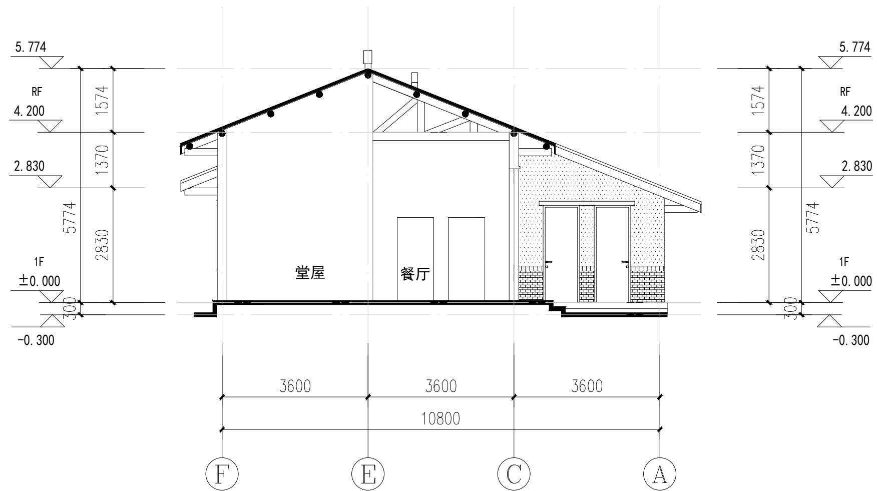
1-1剖面图 1:100
