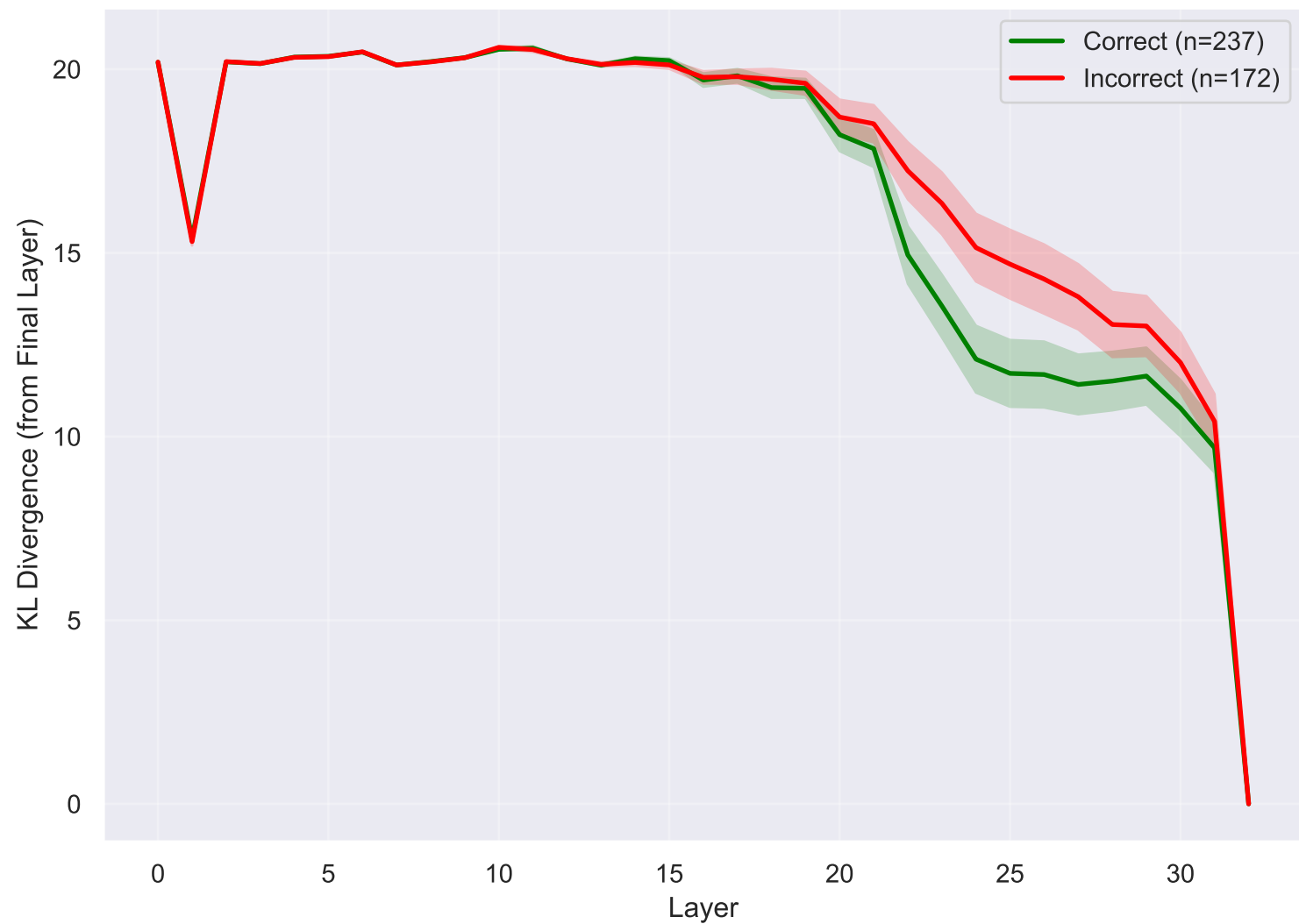
KL Divergence Trajectory - English
