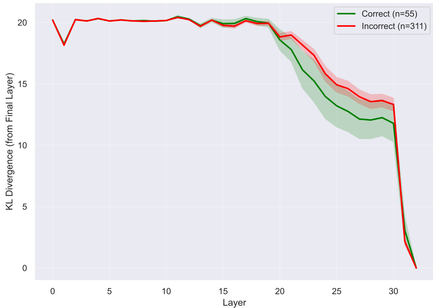
KL Divergence Trajectory - Assamese
