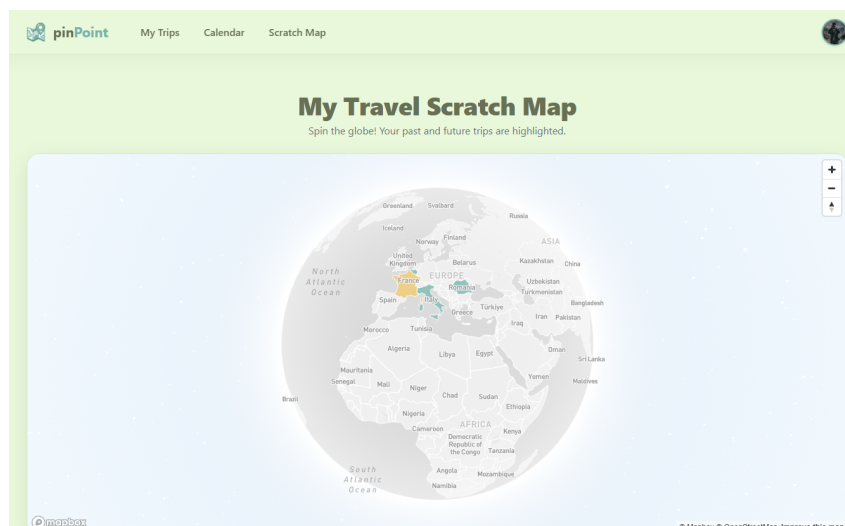
Figura 3.5: Harta interactivă
