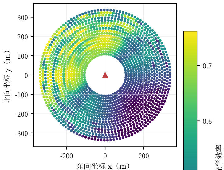
(d) 6月21日 12:00 综合光学效率
