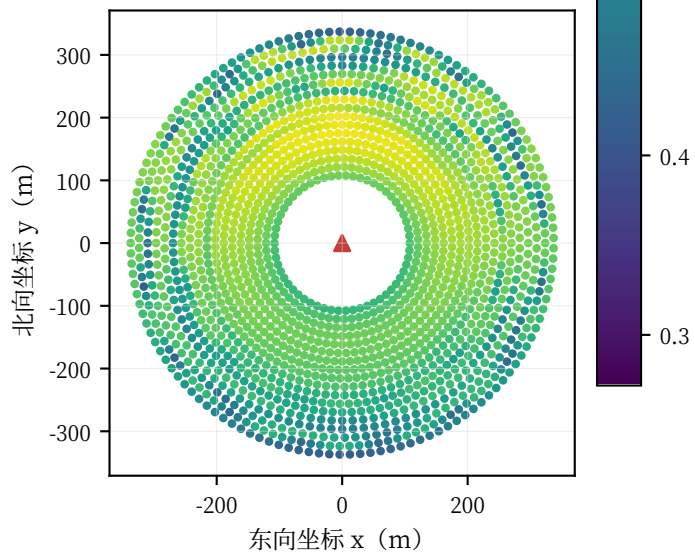
(d) 6月21日 12:00 综合光学效率
