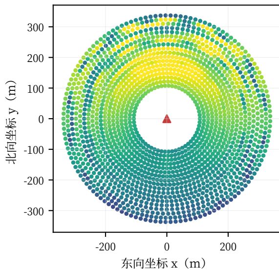
(c) 3月21日 12:00 综合光学效率
