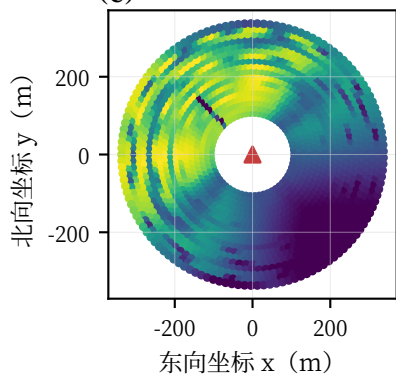
(c) 1月21日 9:00 综合光学效率
