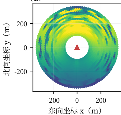
(d) 3月21日 12:00 综合光学效率
