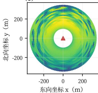
(e) 6月21日 12:00 综合光学效率
