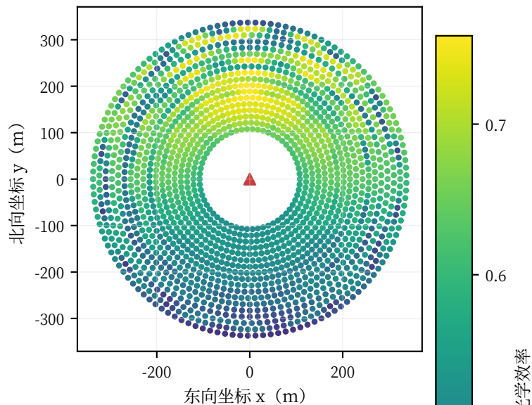
(b) 60个规定状态平均 年均综合光学效率
