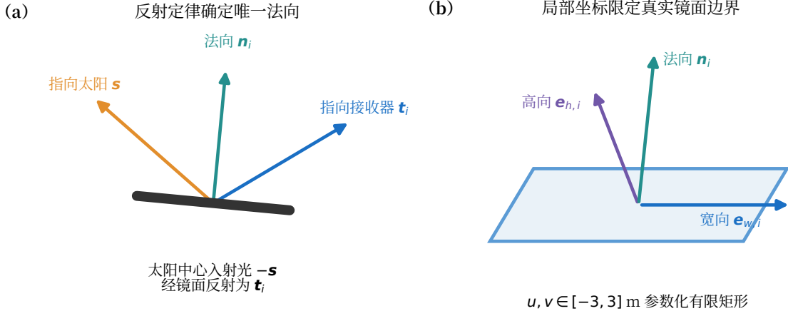
图5 镜面反射方向、唯一法向与有限矩形局部坐标
