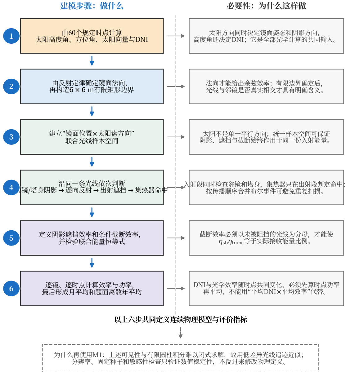
图1 问题一各建模步骤、采用原因及数值求解边界
