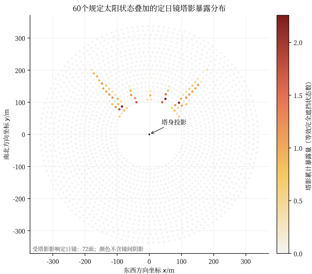
图 10 60 个规定太阳状态叠加的定日镜塔身阴影暴露分布
