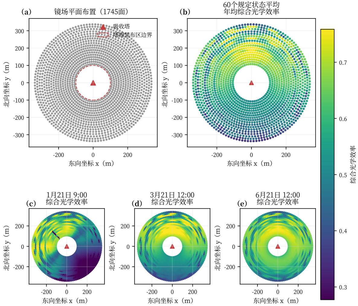
图9 镜场布置、逐镜年均综合光学效率与三个代表状态的逐镜综合光学效率
