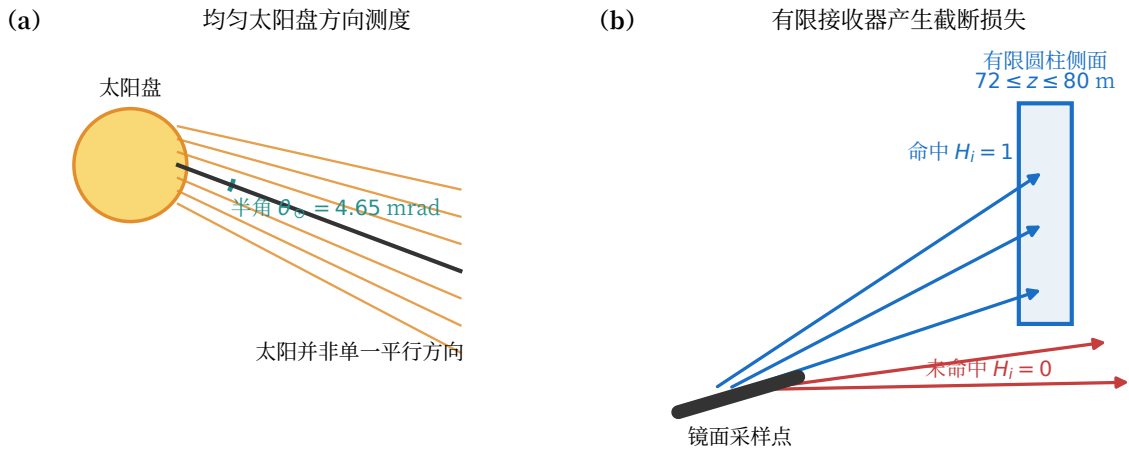
图 7 均匀太阳盘方向与有限圆柱集热器的截断机制
