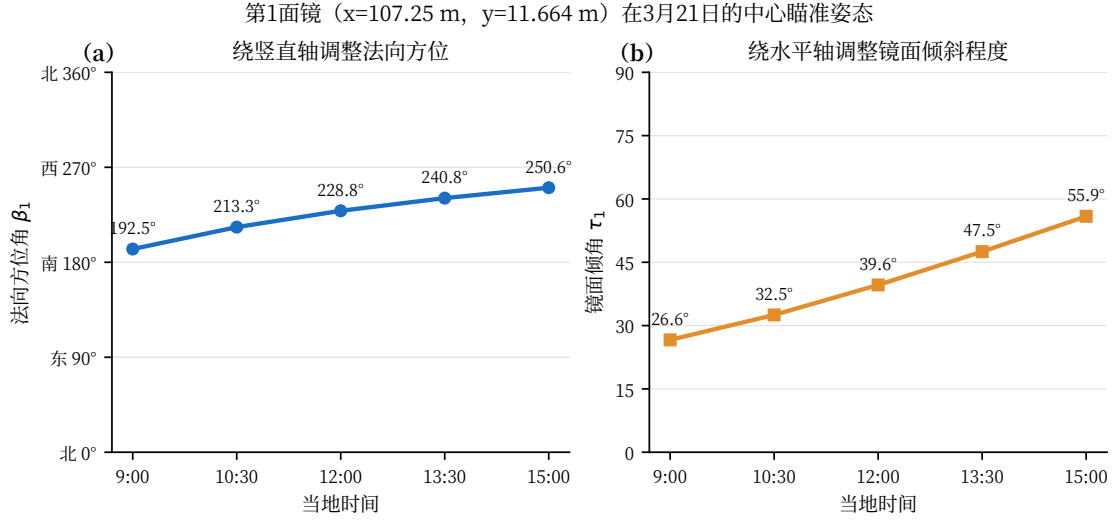
图 4 附件第 1 面定日镜在 3 月 21 日的时变目标姿态
