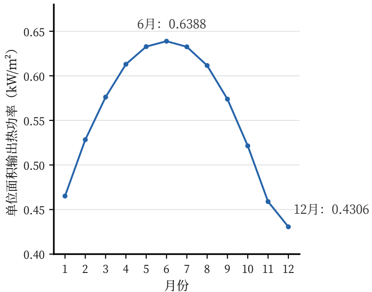
(b) 单位镜面面积月平均输出热功率
