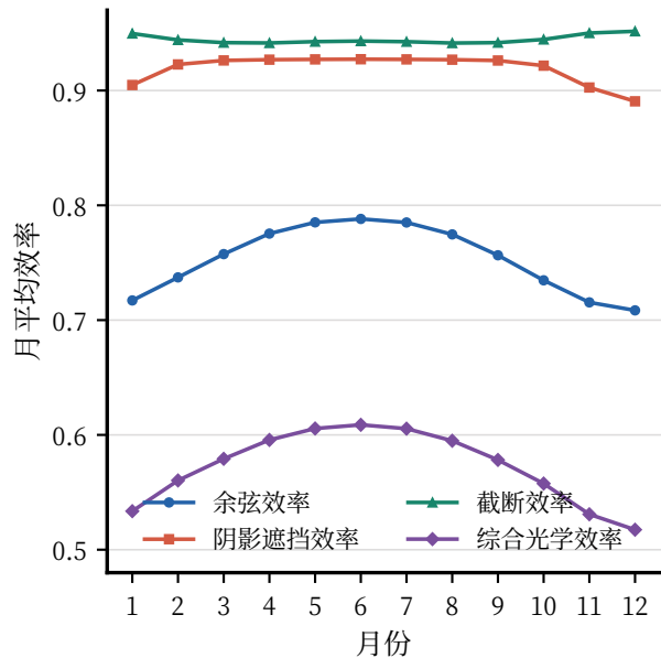
(a) 月平均光学效率分解
