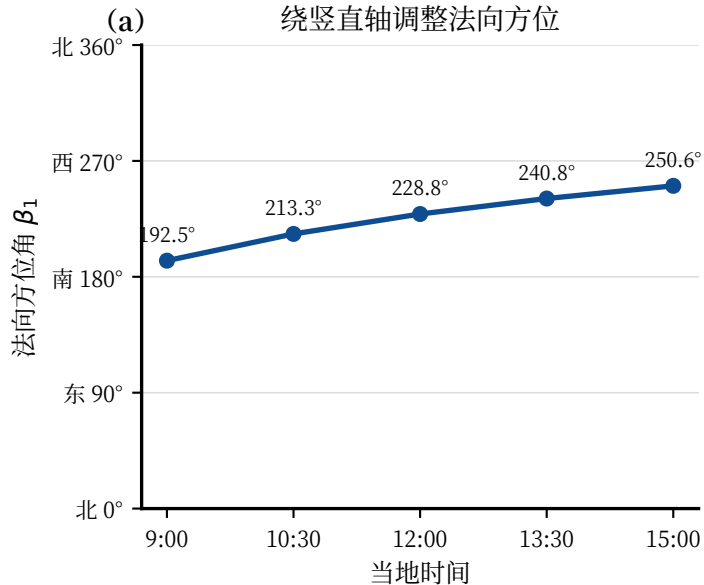
第1面镜 (x=107.25 m, y=11.664 m) 在3月21日的中心瞄准姿态
