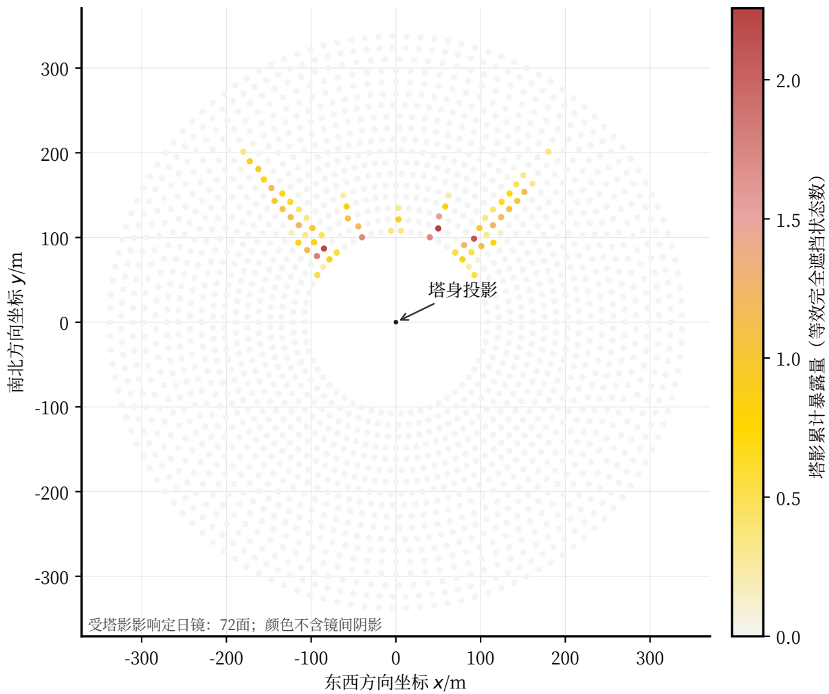
60个规定太阳状态叠加的定日镜塔影暴露分布
