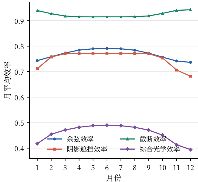
(a) 月平均光学效率分解
