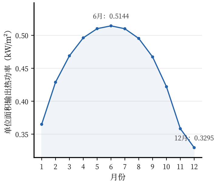
(b) 单位镜面面积月平均输出热功率
