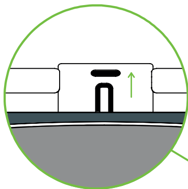
Encaixe superior através de sistema HOOK MGB
