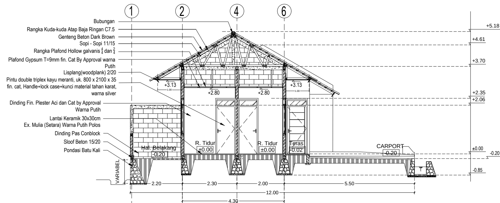
A Potongan - 3 A-03-07 Skala 1:100
