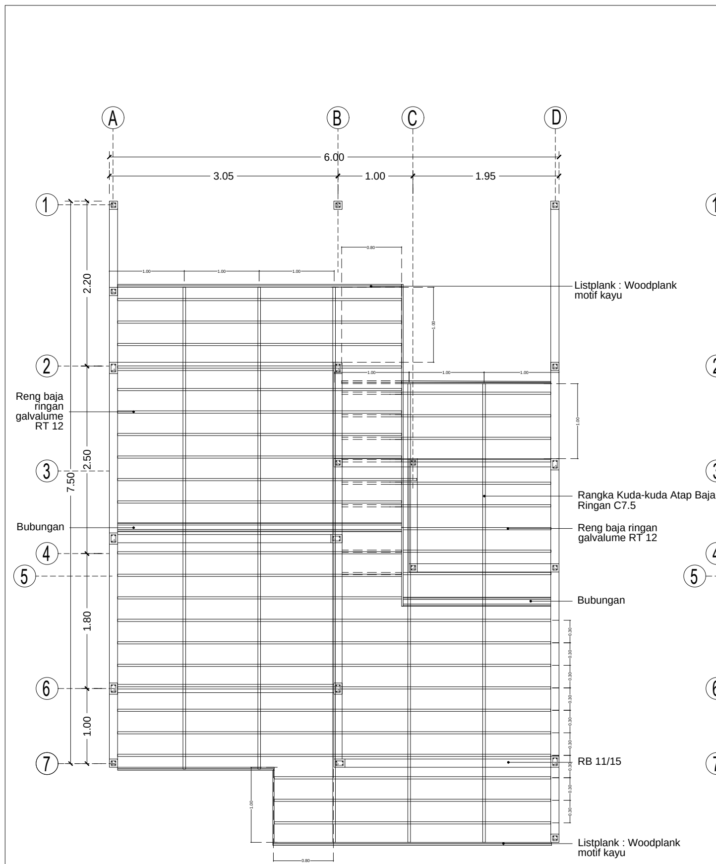
DENAH RENCANA ATAP
