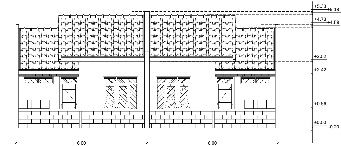
A Tampak - B A-02-05 Skala 1:100
