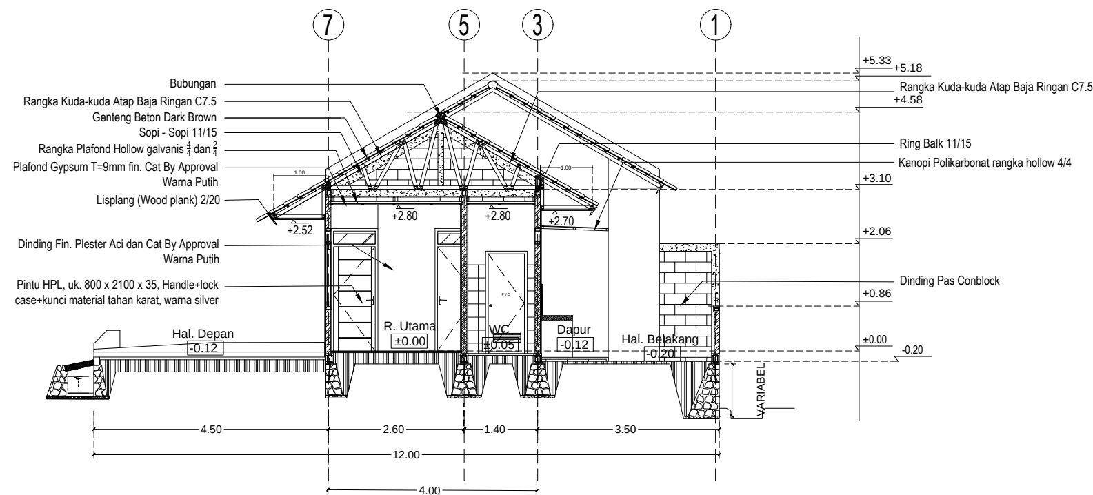
A Potongan - 4 A-03-07 Skala 1:100
