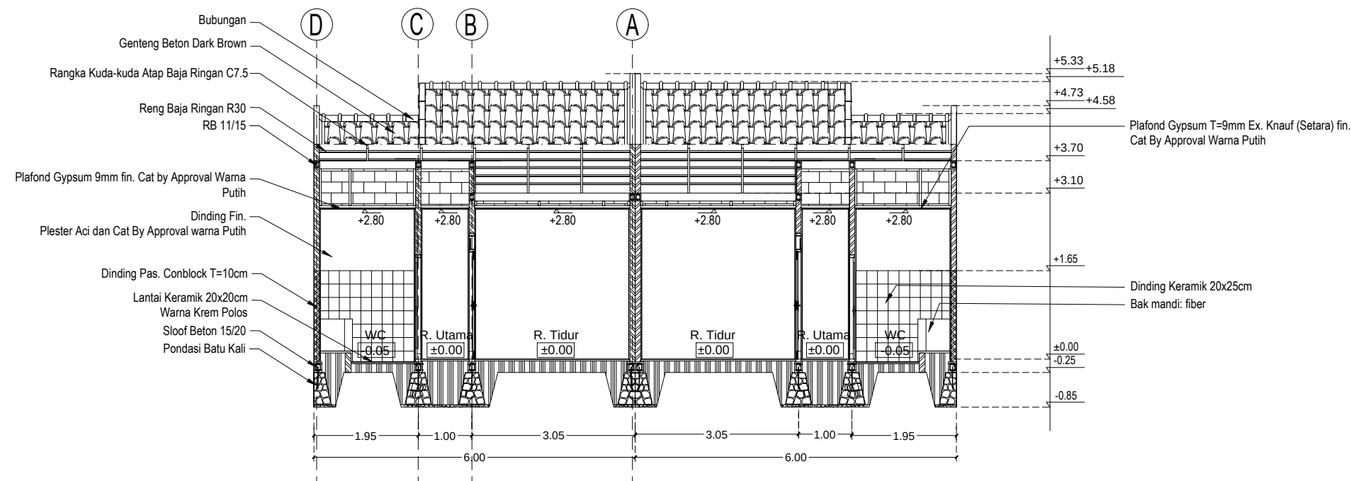
A Potongan - 2 A-03-06 Skala 1:100
