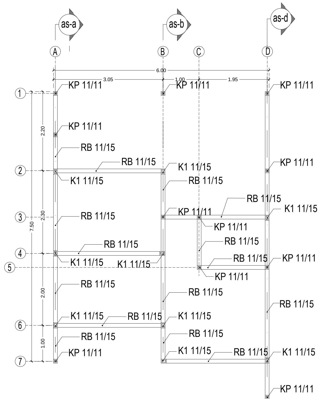
DENAH RENCANA PORTAL Skala 1:50
