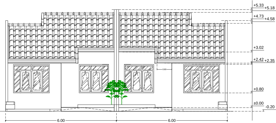
A Tampak - A A-02-05 Skala 1:100
