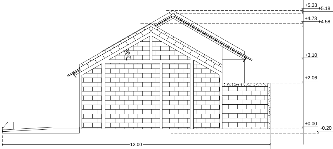
A Tampak - D A-02-05 Skala 1:100
