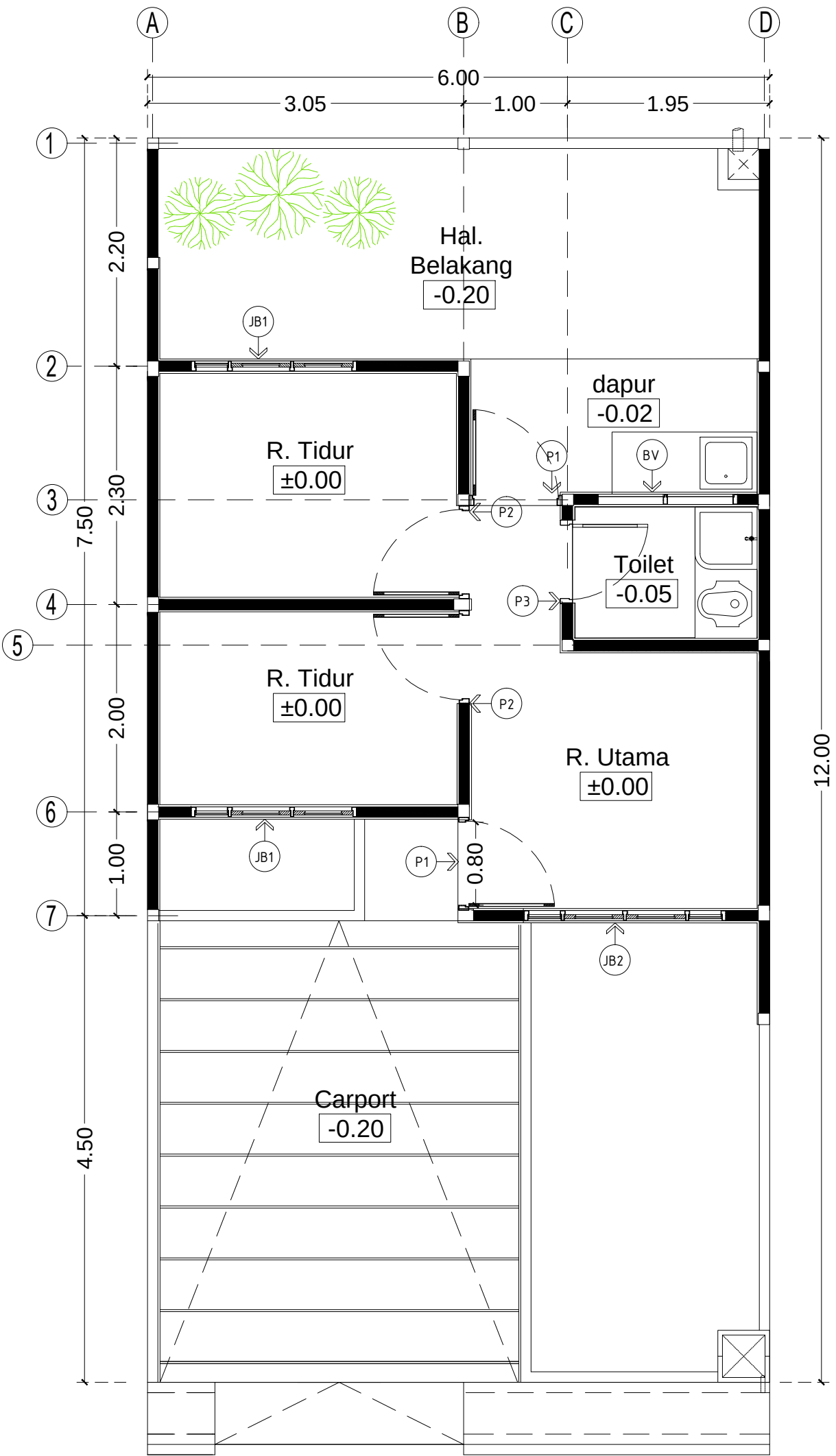
Denah Rencana Kusen
