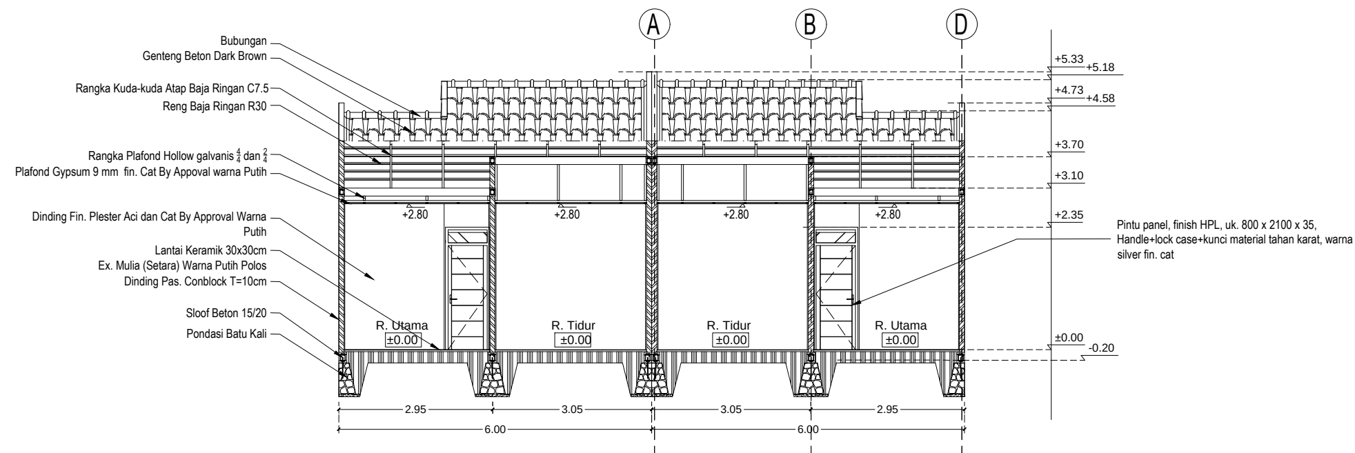
A Potongan - 1 A-03-06 Skala 1:100
