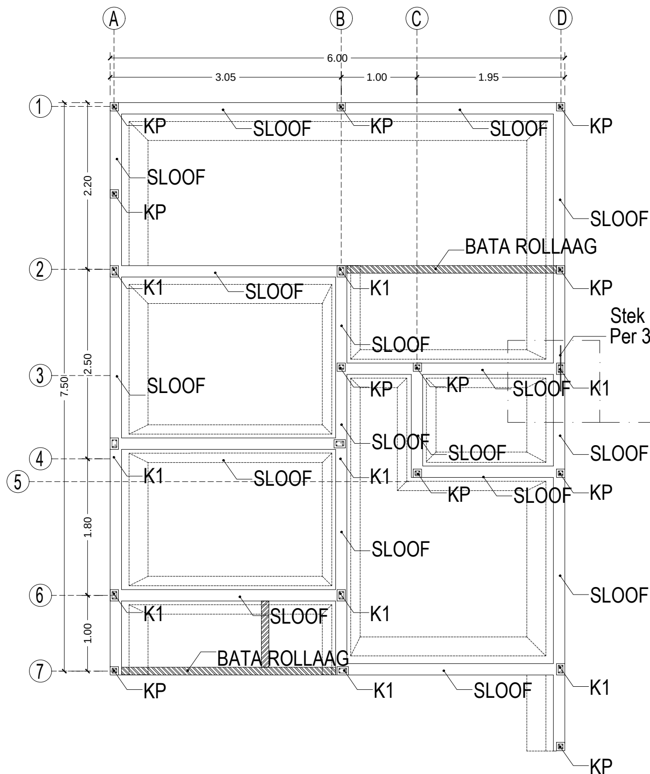
DENAH RENCANA PONDASI Skala 1:50
