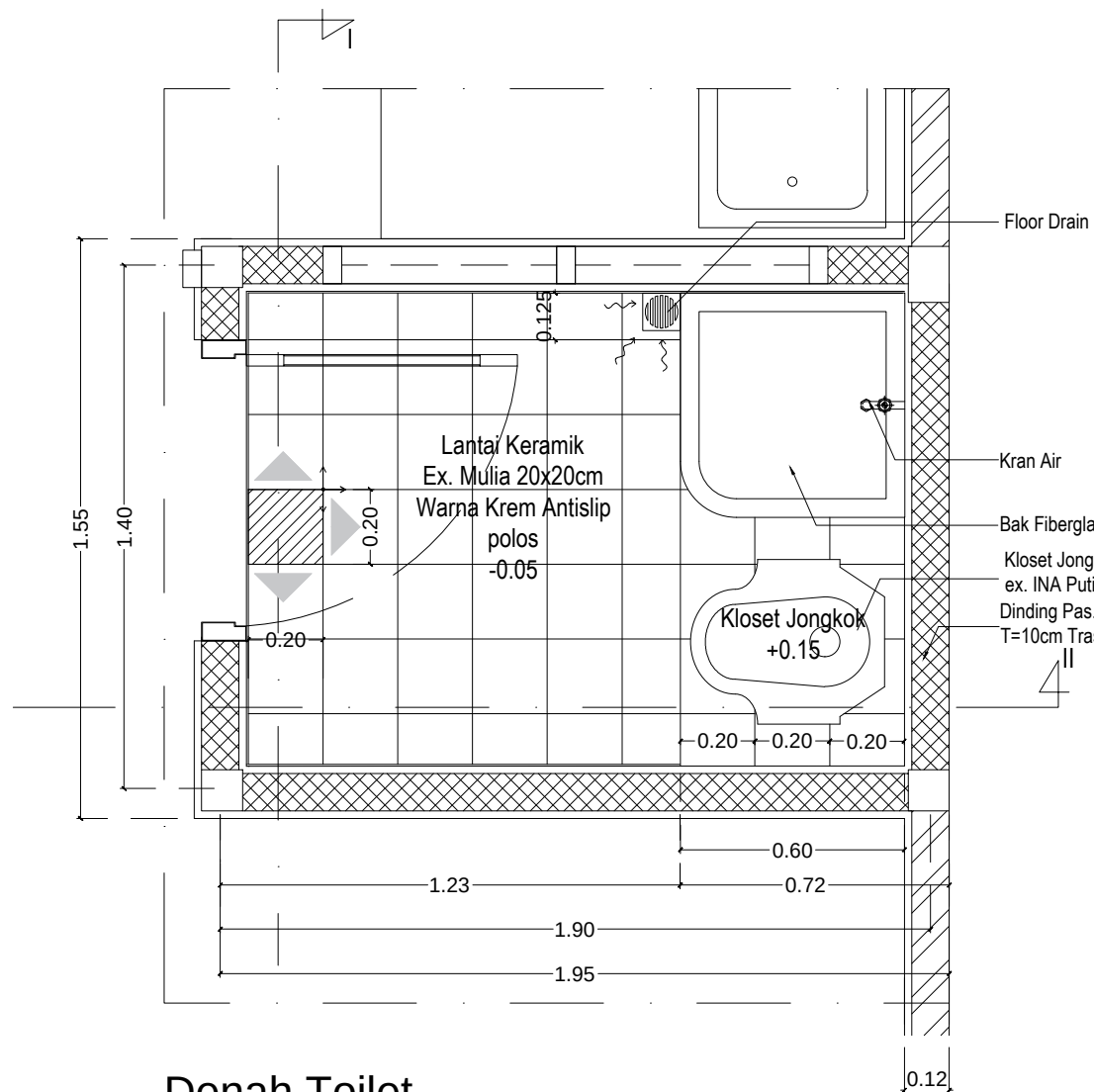
Denah Toilet
