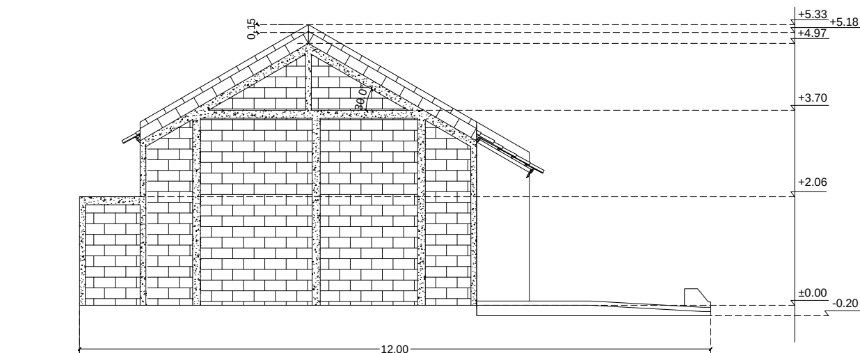
A Tampak - C A-02-05 Skala 1:100
