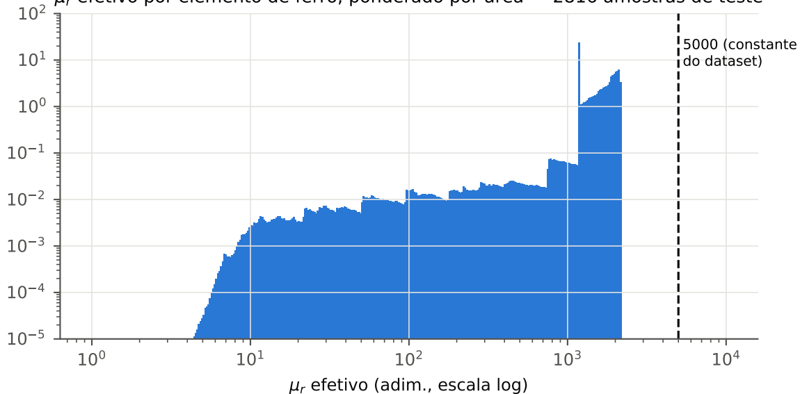
\mu_r efetivo por elemento de ferro, ponderado por área — 2816 amostras de teste
