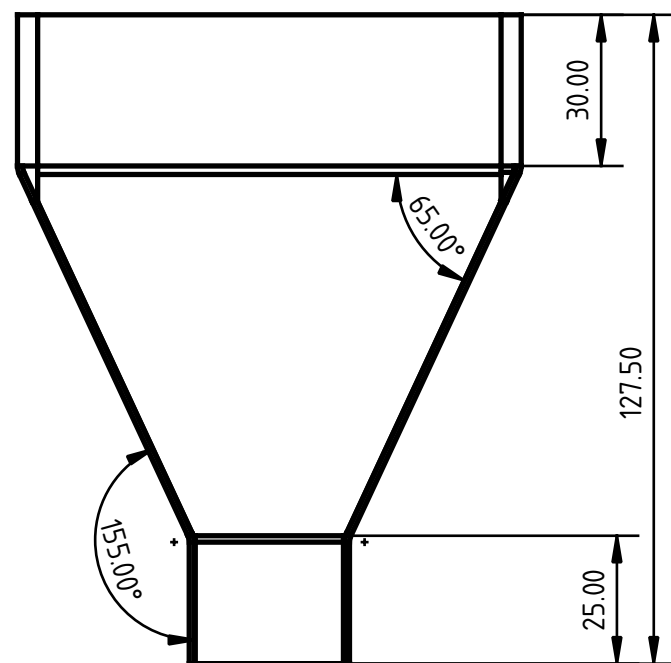
正面図 (Front View)
