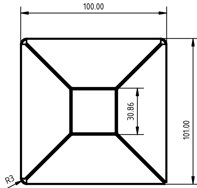
上面図 (Top View)
