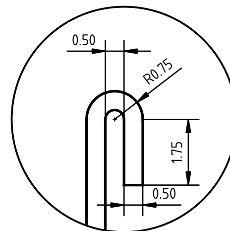
詳細 1 (DETAIL 1) (10 : 1)
