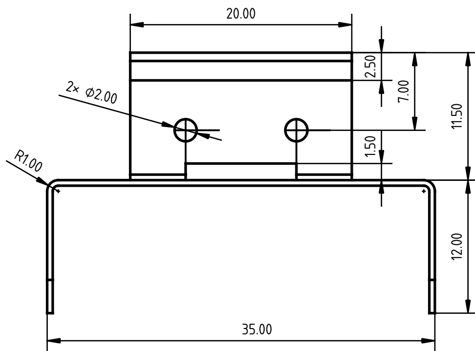
正面図 (FRONT VIEW)
