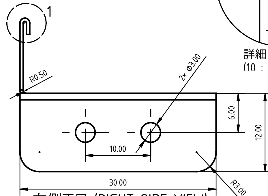
右側面図 (RIGHT SIDE VIEW)
