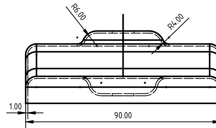
背面図(REAR VIEW)
