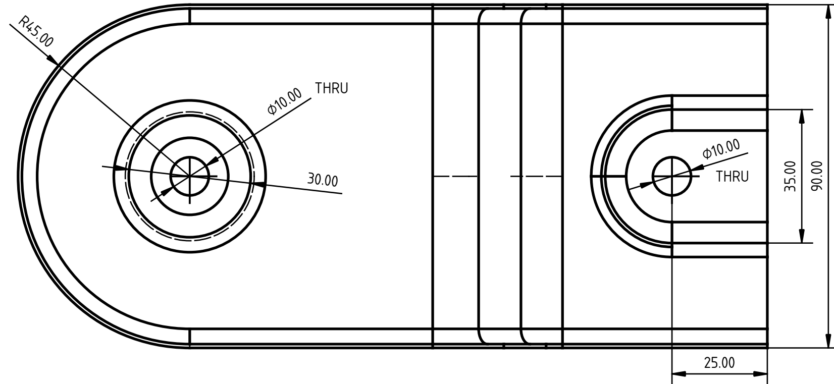
上面図(TOP VIEW)
