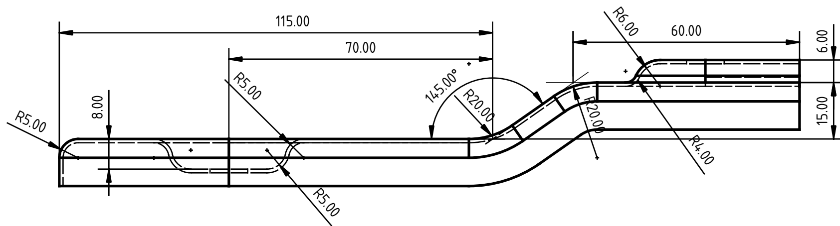
右側面図(TOP RIGHT VIEW)
