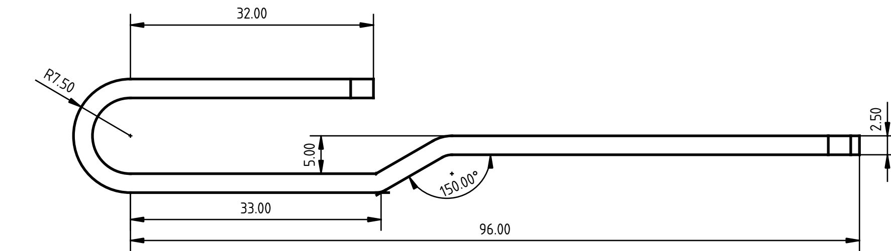
正面図(FRONT VIEW)
