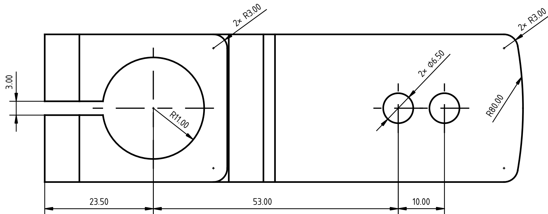
上面図(TOP VIEW)
