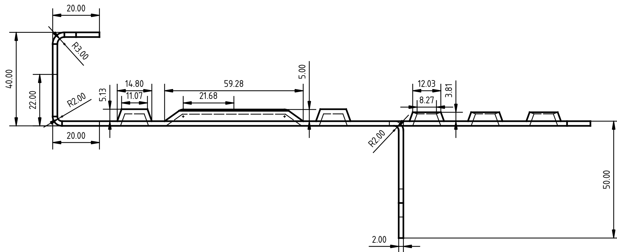
正面図(FRONT VIEW)
