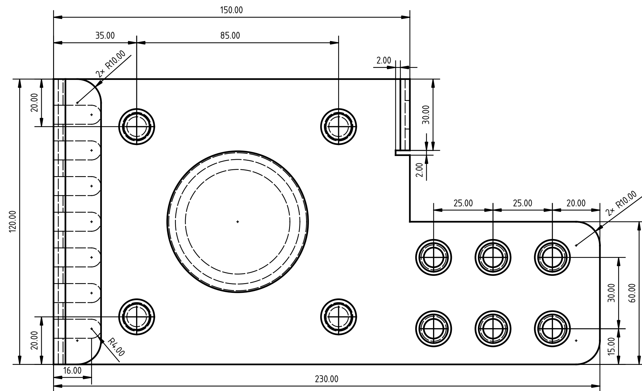
上面図(TOP VIEW)
