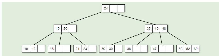
Figure 3.4: Árbol B
